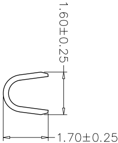
SEC:B-B
